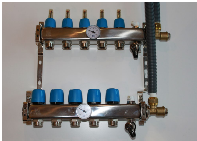
Bild 2. Anslutning mot Värmekretsfordelaren.
