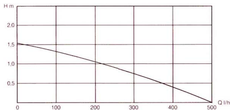
Kapacitetsdiagram LK-KrePu
