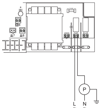
Kopplingschema inkoppling av pump
