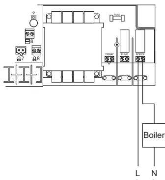
Kopplingschema inkoppling av värmekälla
