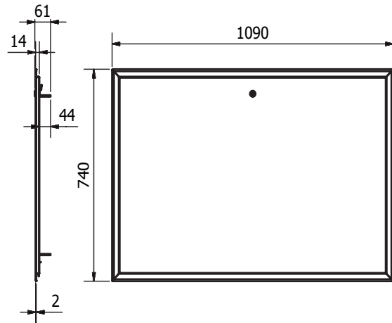
LK Frame/hatch UFH 1050, INB
