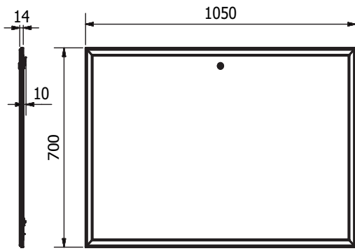
LK Frame/hatch UFH 1050, UTV
