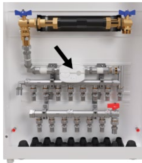
Vedenalvontayksikkö asennettuna kaappiin.
