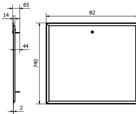
LK Frame/hatch UFH 1050 INB
