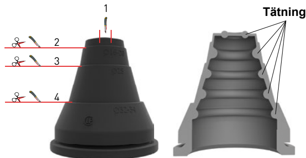
Kapning av rör genomföring.
