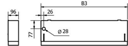
LK Sockel
