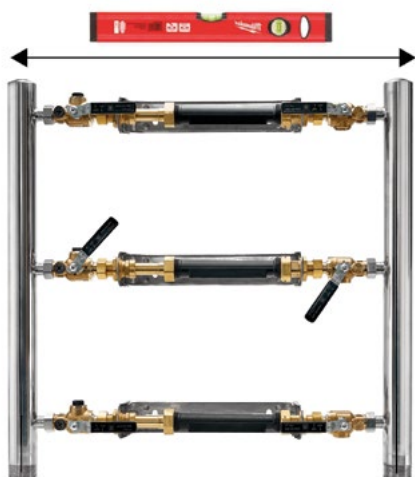
Bilden visar LK PVK med ett vattenmått för horisontell montering.
