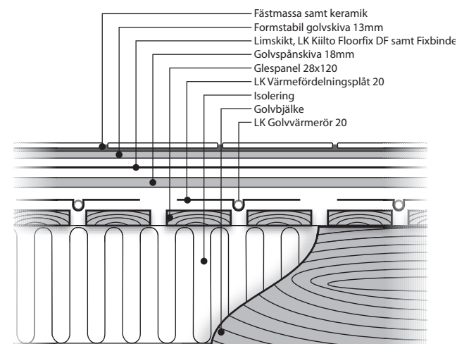
Värmefördelningsplåt 20 monterat i glespanel på golvbjälkar. Keramiskt ytskikt i torra utrymmen.
