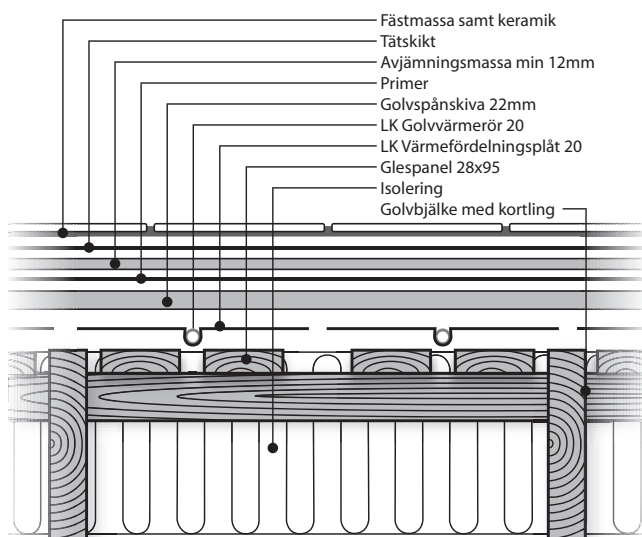
Värmefördelningsplåt 20 monterat i glespanel mellan golvbjälkar. Keramiskt ytskikt i våta utrymmen.
