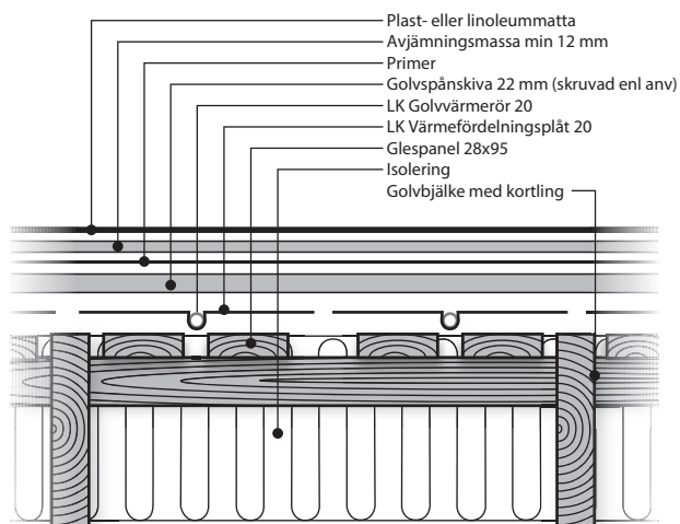
Värmefördelningsplåt 20 monterat i glespanel mellan golvbjälkar. Ytskikt plast- eller linoleummatta.
