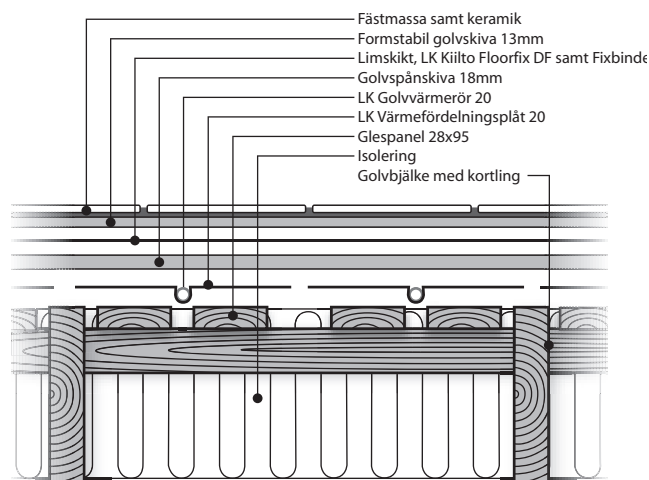
Värmefördelningsplåt 20 monterat i glespanel mellan golvbjälkar. Keramiskt ytskikt i torra utrymmen.
