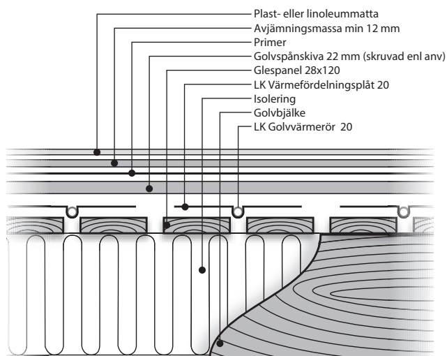
Värmefördelningsplåt 20 monterat i glespanel på golvbjälkar. Ytskikt plast- eller linoleummatta.
