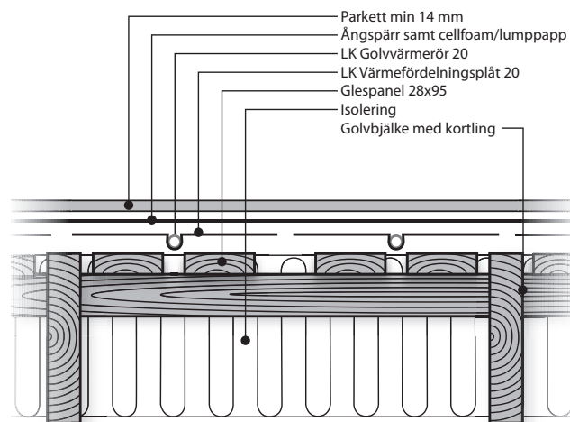
Värmefördelningsplåt 20 monterat i glespanel mellan golvbjälkar. Ytskikt parkett.
