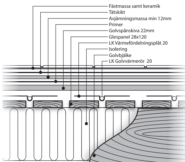
Värmefördelningsplåt 20 monterat i glespanel på golvbjälkar. Keramiskt ytskikt i våta utrymmen.
