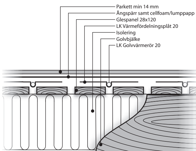
Värmefördelningsplåt 20 monterat i glespanel på golvbjälkar. Ytskikt parkett.
