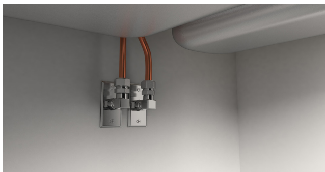
När genomföring av LK PE-X och PAL Universälör RiR utan väggdosa skall ansluta till t.ex. köks- eller tvättställsblandare, skall vinkeln i övergång mellan LK PE-X–LK PAL rör och blandarens anslutningsrör fixeras. Detta sker förslagsvis med väggbrička försedd med gänganslutning.
