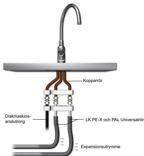
Godtagbar lösning vid installation av köksblandare med anslutningsrör av koppar med LK PE-X och PAL Universalsrör RiR.
