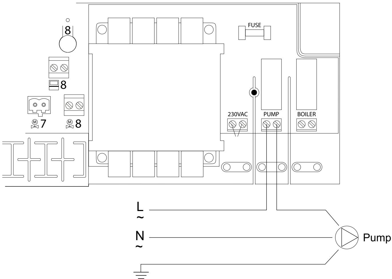
Kopplingsschema för inkoppling av pump till mottagar-enhet 8.
